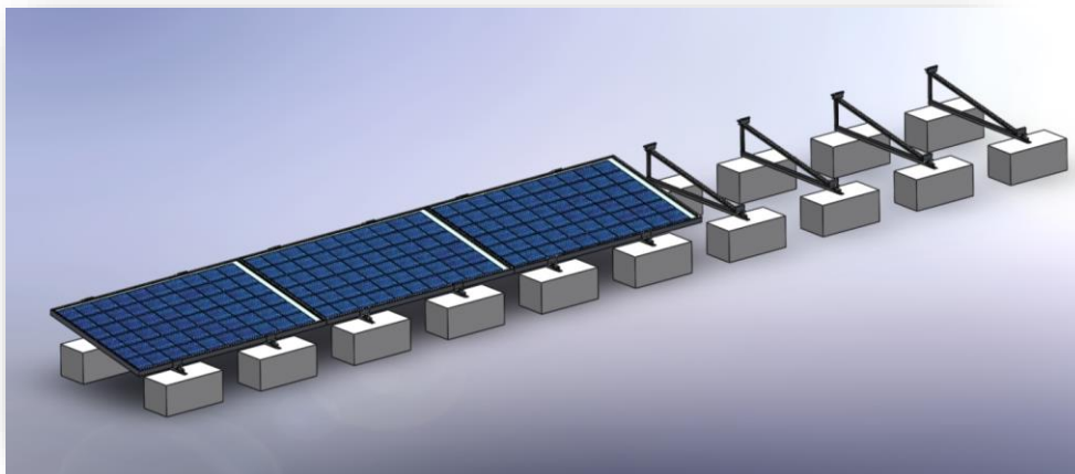
2. ΤΡΙΓΩΝΙΚΟ ΣΥΣΤΗΜΑ ΣΤΗΡΙΞΗΣ
