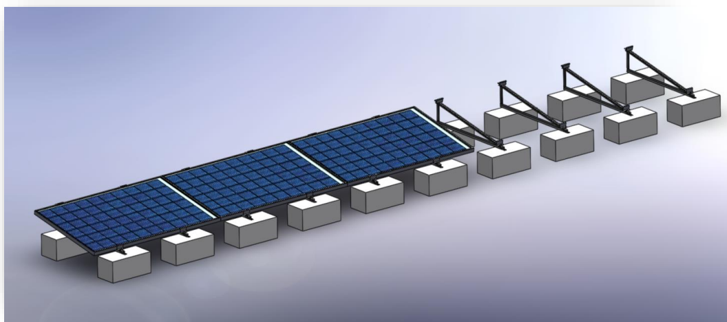
2. ΠΡΟΣΥΝΑΡΜΟΛΟΓΗΜΕΝΟ ΤΡΙΓΩΝΟ
