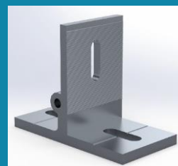
4.ΠΕΛΜΑ
