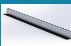
3.ΠΟΔΙ
